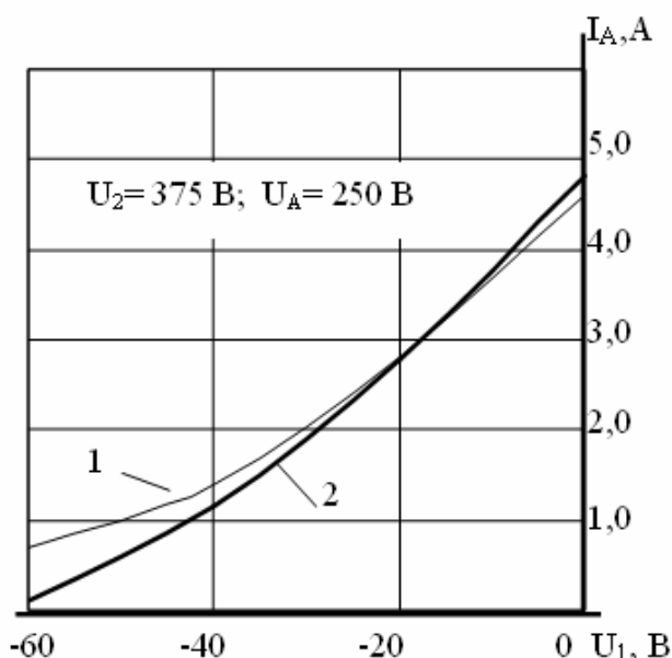
Рисунок 2 – Анодно-сеточные характеристики: 1 – по паспортным данным; 2 – полученные расчетом
