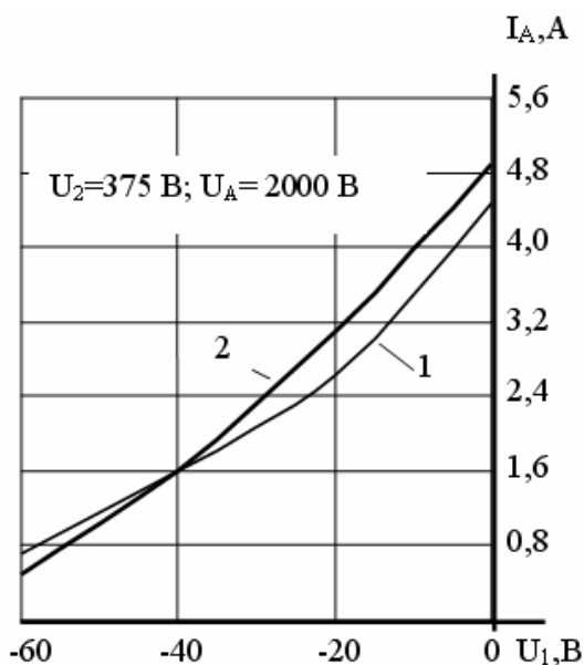
Рисунок 1 – Анодно-сеточные характеристики: 1 – по паспортным данным; 2 – полученные расчетом
